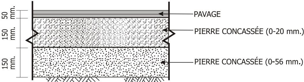
Figure 1 : Pavage et fondation – Coupe type
